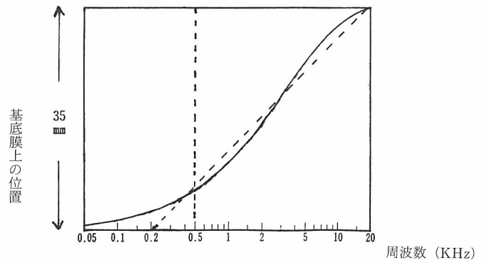
図5 音の大きさ、高さの感覚が対数的であることの説明
