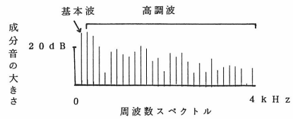
ギター音とその成分音
