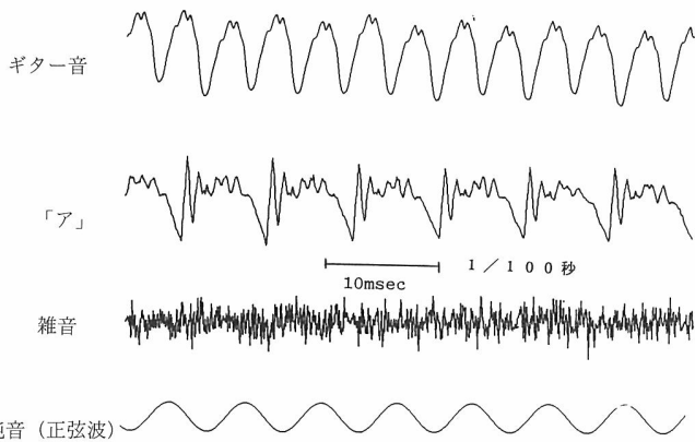
図2 様々な音の波形、上からギター音、音声「ア」、雑音、純音
