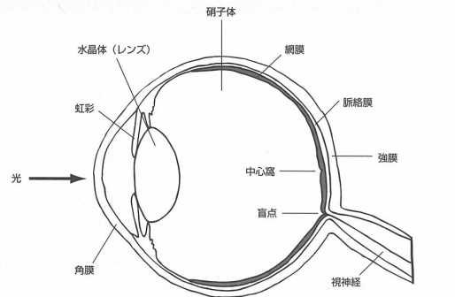
図 3.10 眼球の構造
